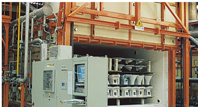
Four à sole mobile dans l'industrie de la céramique
